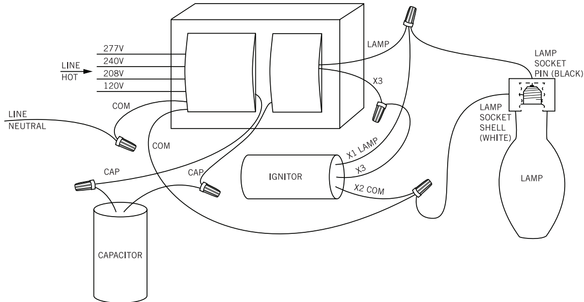
HID WIRING DIAGRAM: H3
